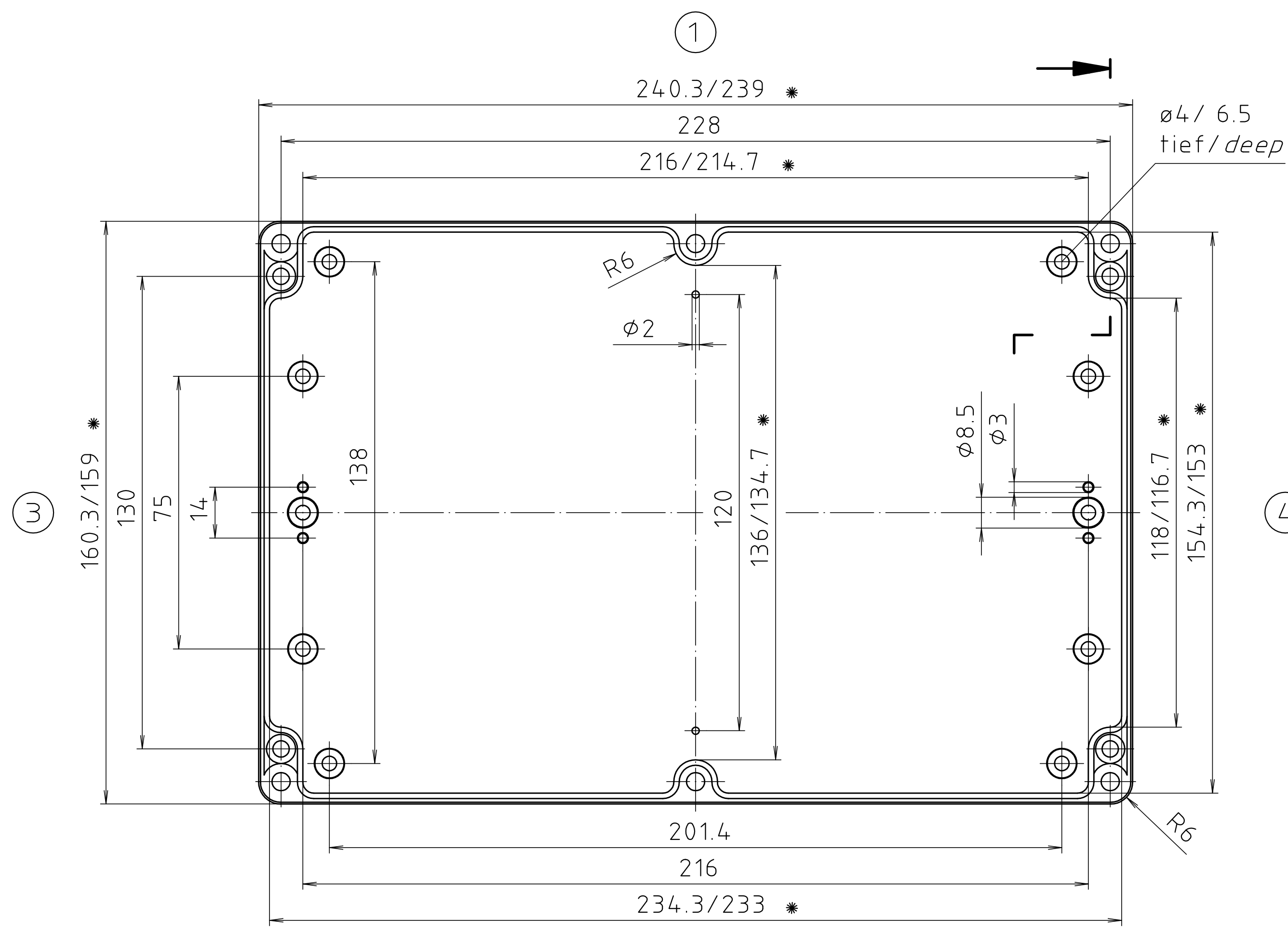
Unterteil/base
