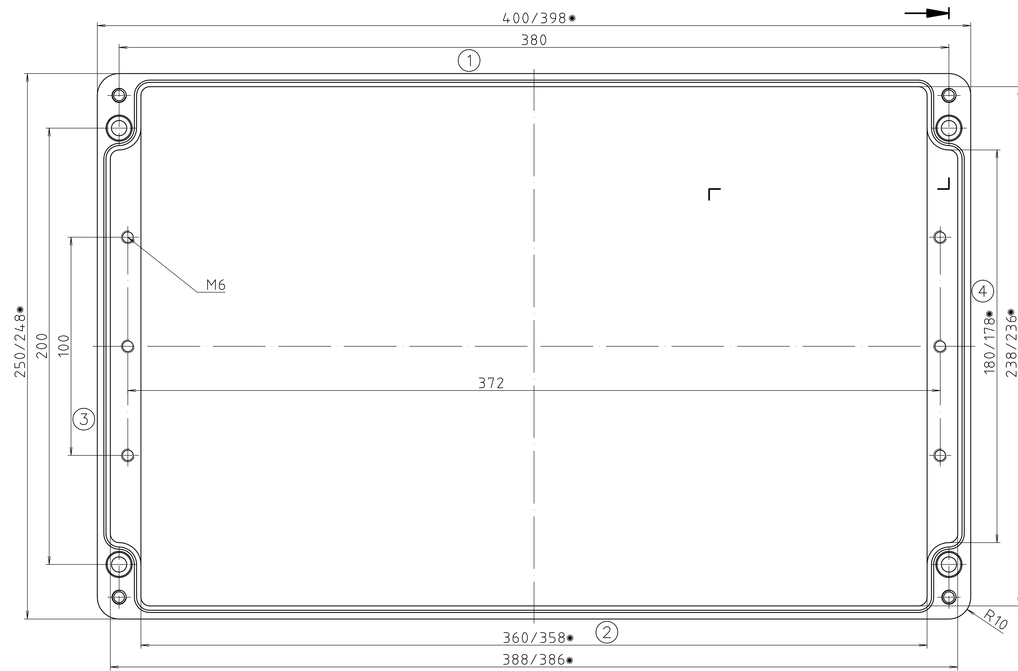
Unterteil/ base
