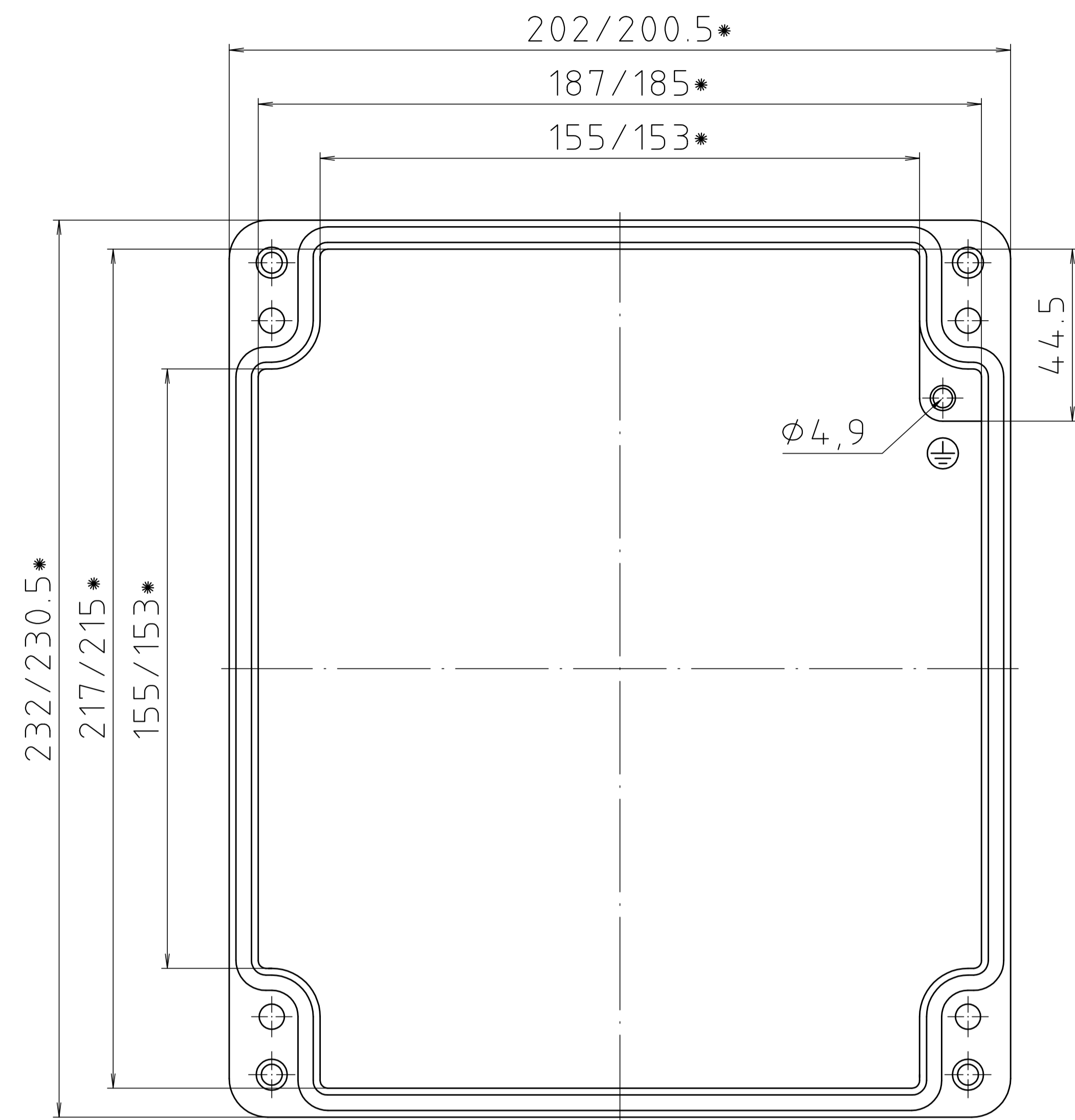
Deckel / lid
