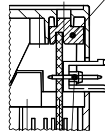
Stiffleiste STL 950/___ V/ pin bars STL 950/___ V
