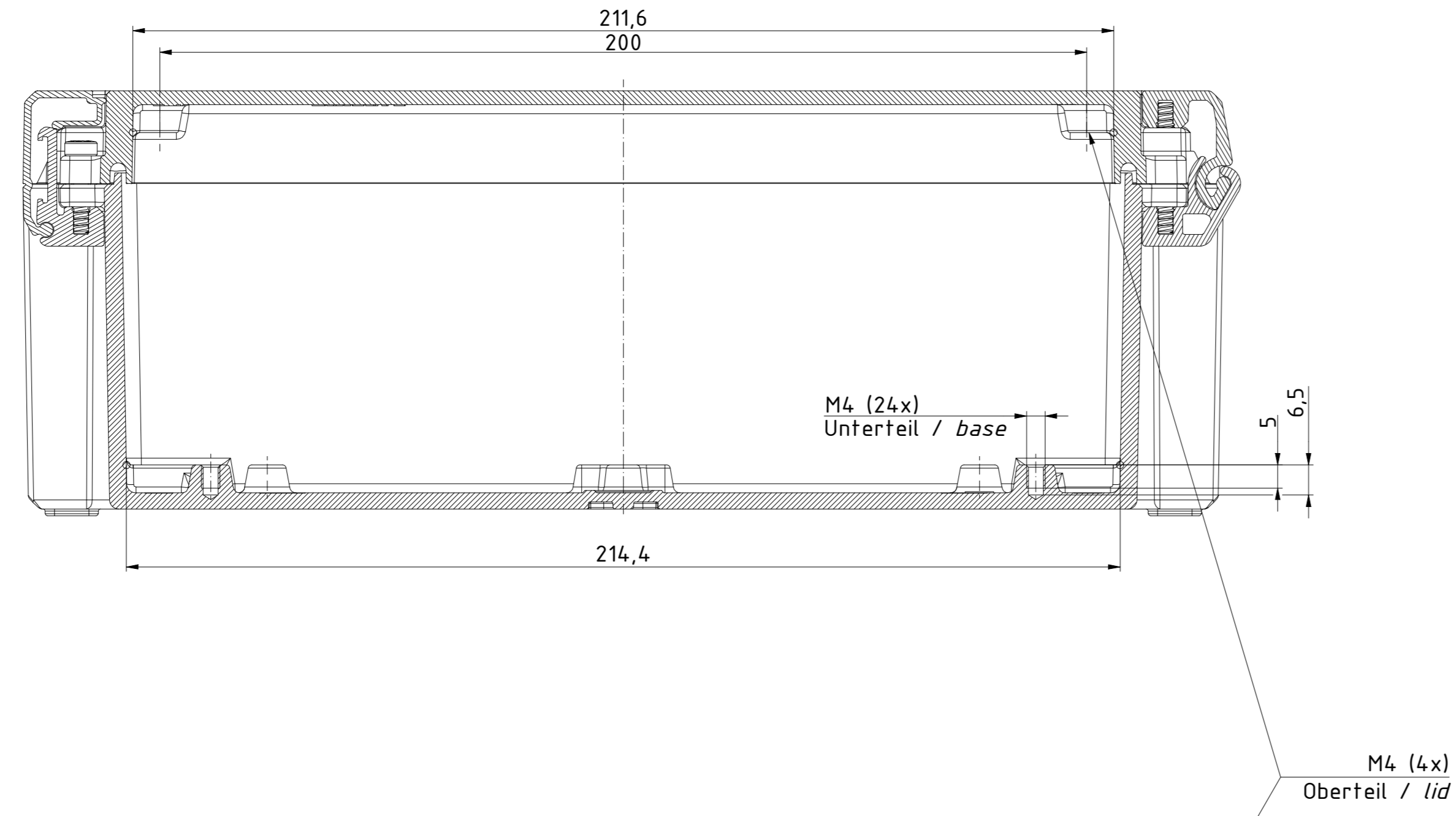
B-B ( 1 : 1 )
