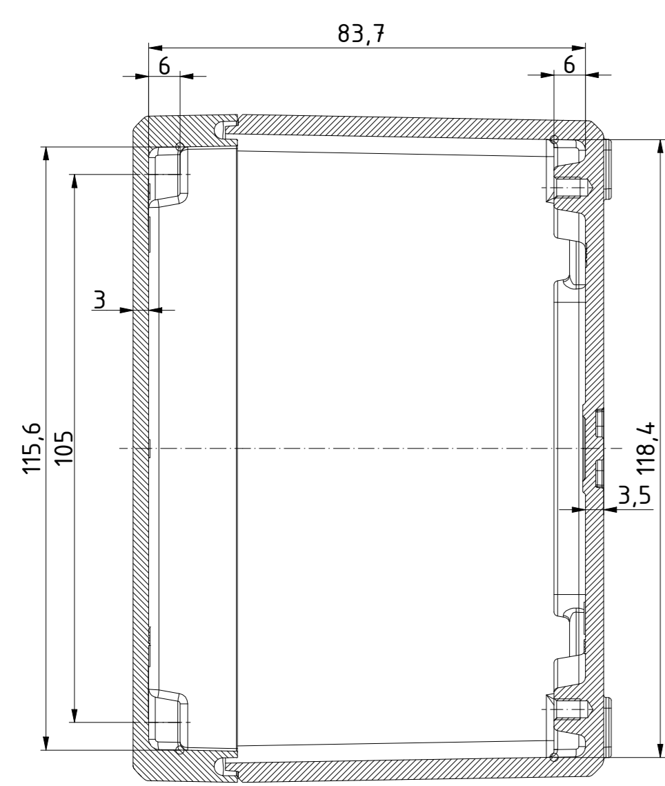
A-A ( 1 : 1 )
