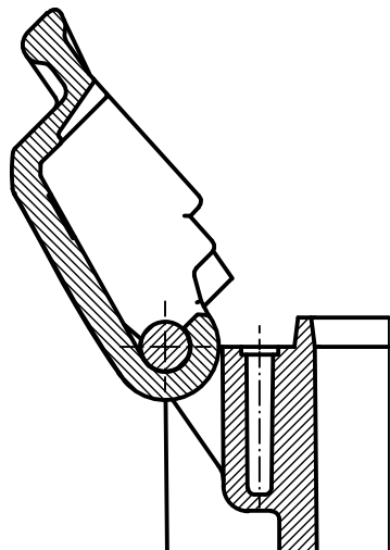
B SC HB-E montiert B SC HB-E mounted
